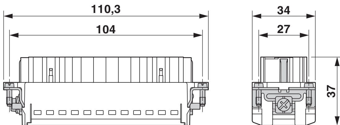
Maßzeichnung
