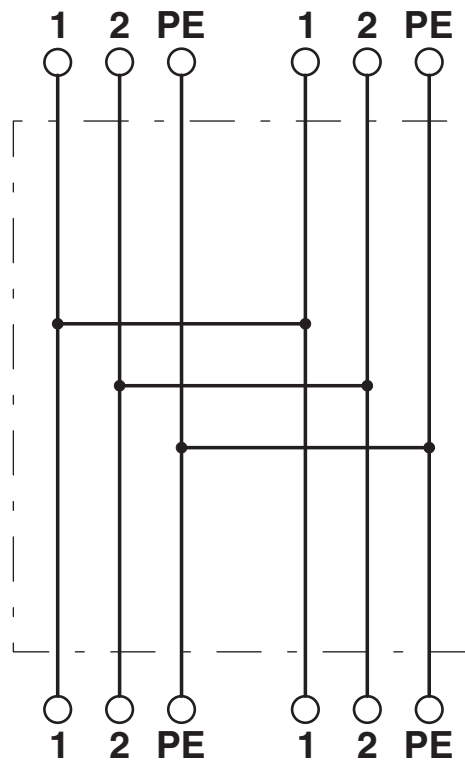
Schaltplan
