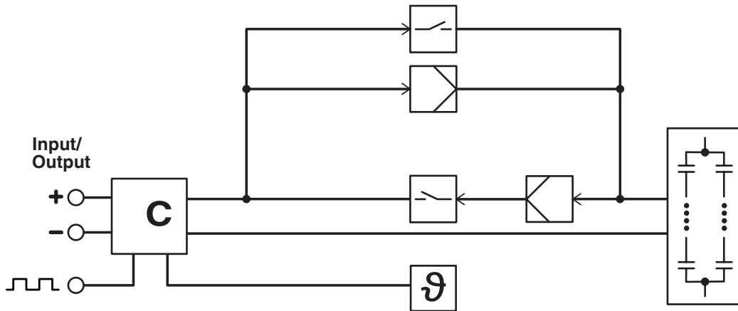
Blockschaltbild
