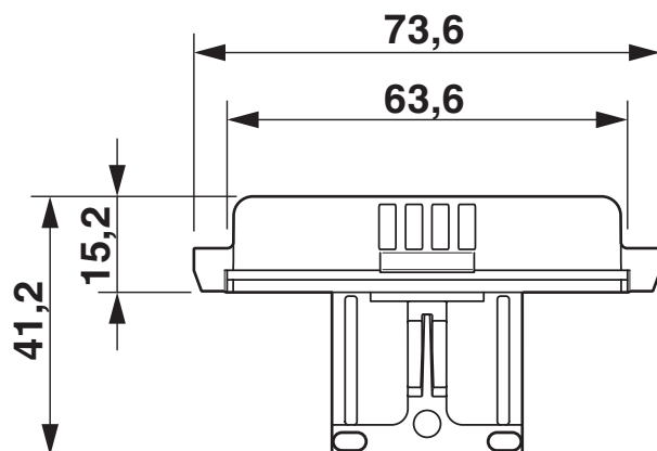
Dessin coté
