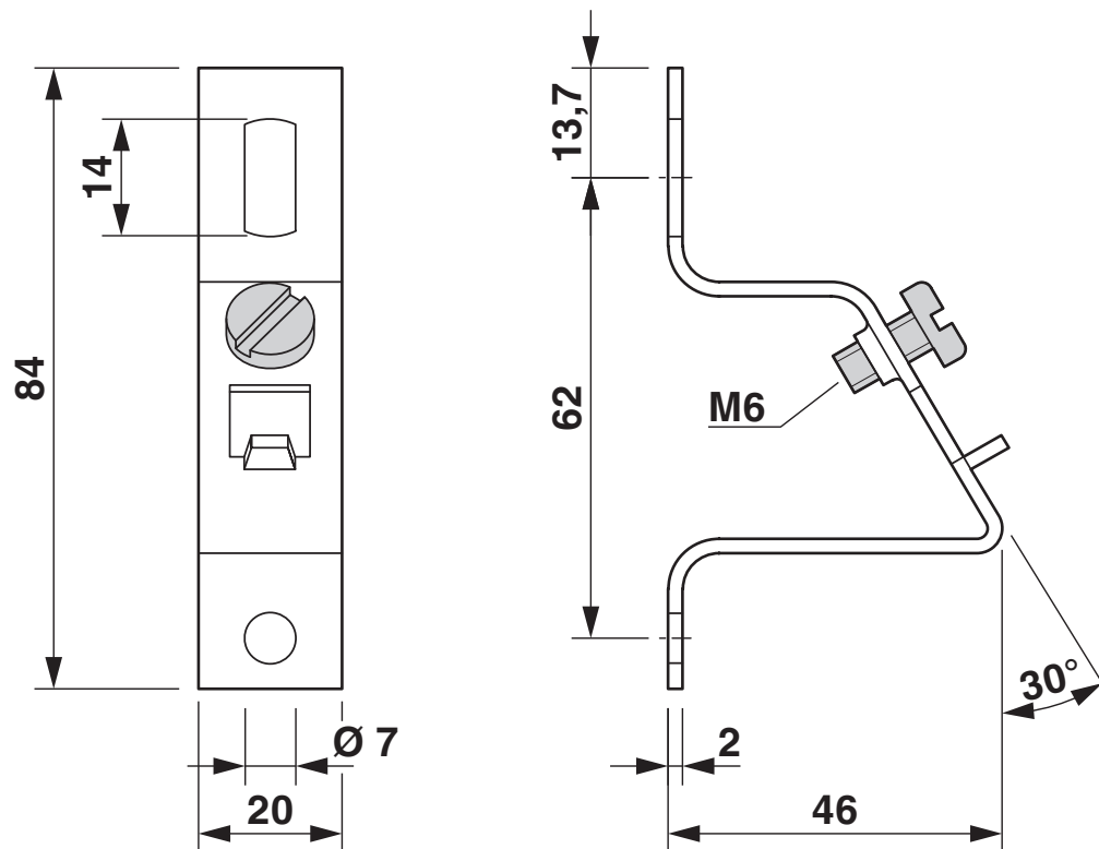
Maßzeichnung
