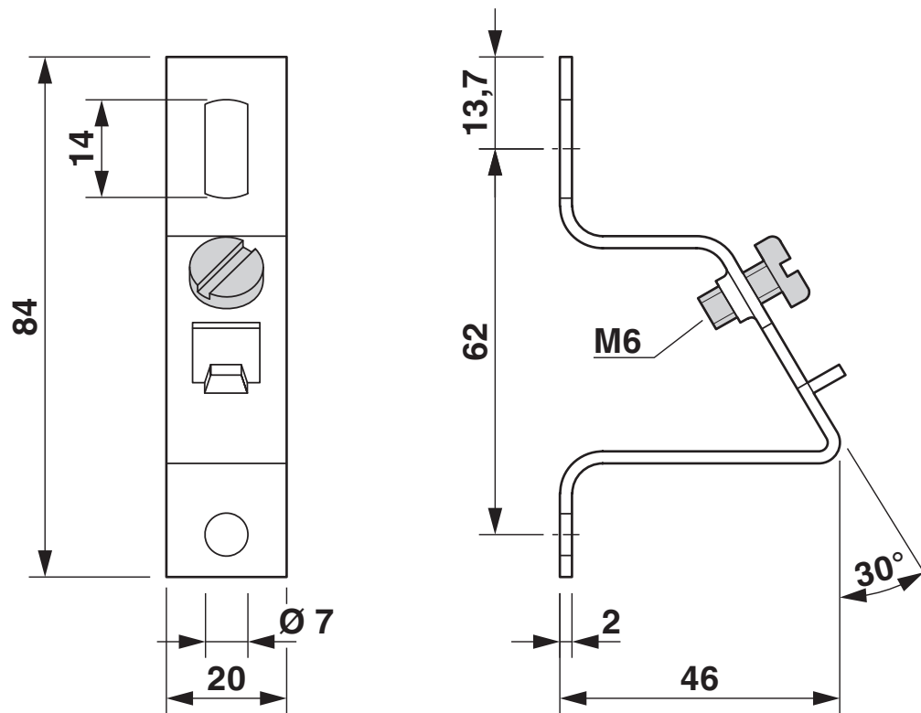
Dessin coté
