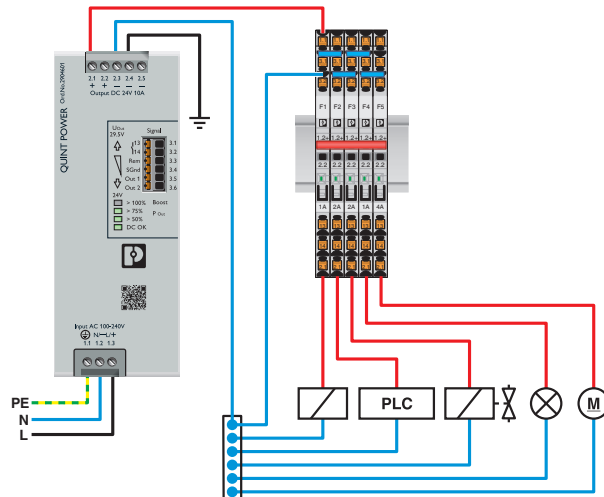
Applikationszeichnung
