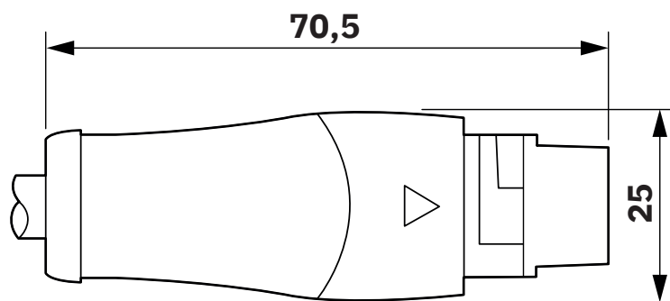
Dessin coté
