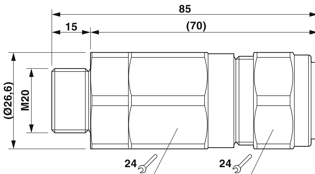
Maßzeichnung
