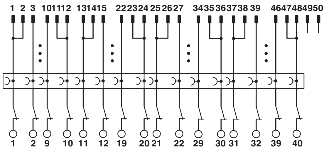
Esquema de conexiones FLKM 50/KDS3-MT/PPA/S7-300
