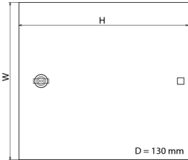
Dimensiones del DPG LSA 220 P
