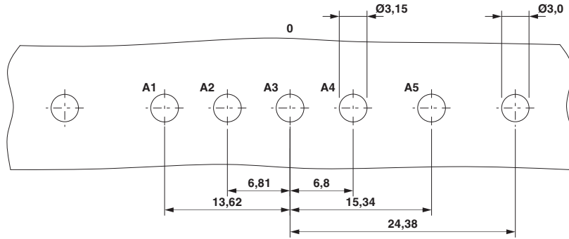
Bohrplan/Lötpadgeometrie
