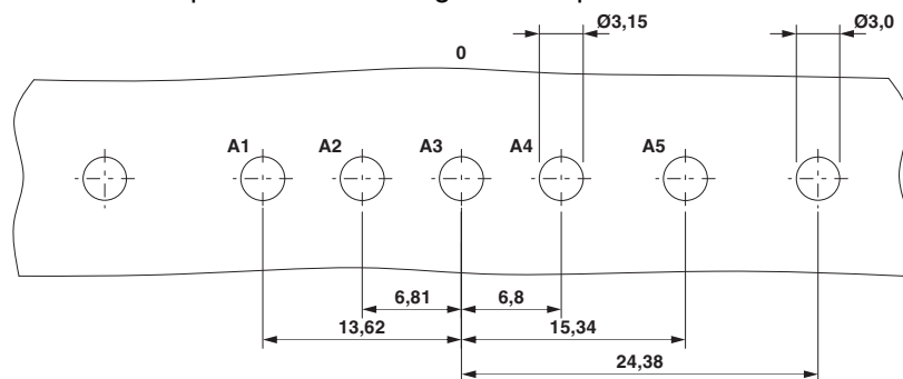
Esquema de taladros/geometría pads soldadura
