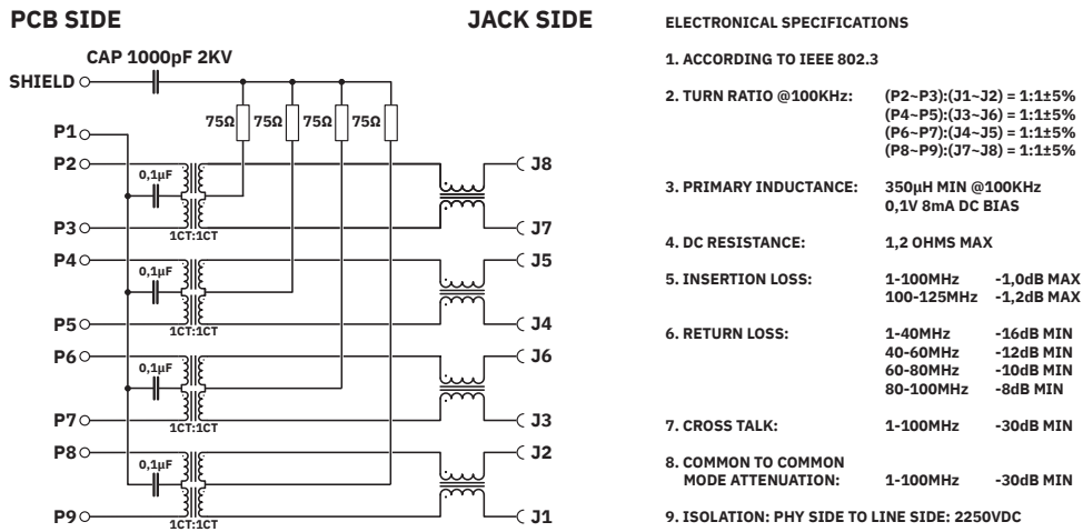
Diagrama eléctrico
