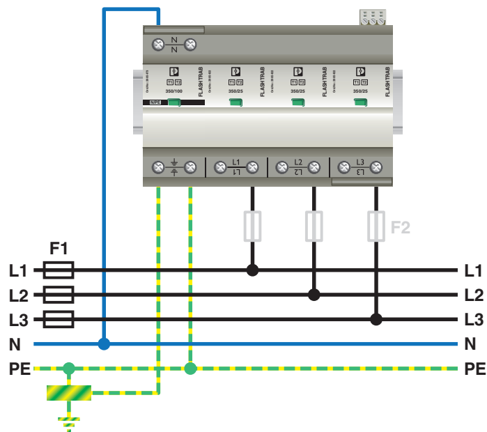
Applikationszeichnung
