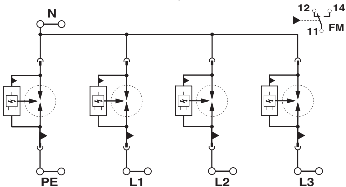
Schaltplan
