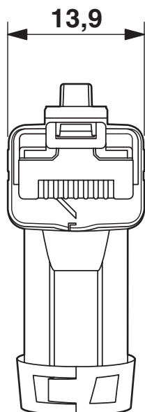
Connecteur mâle RJ45, IP20, coudé
