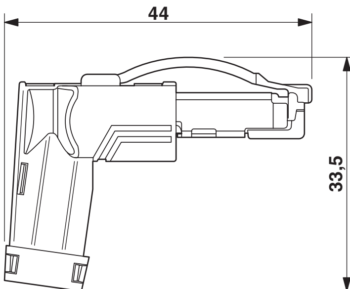
Dessin coté
