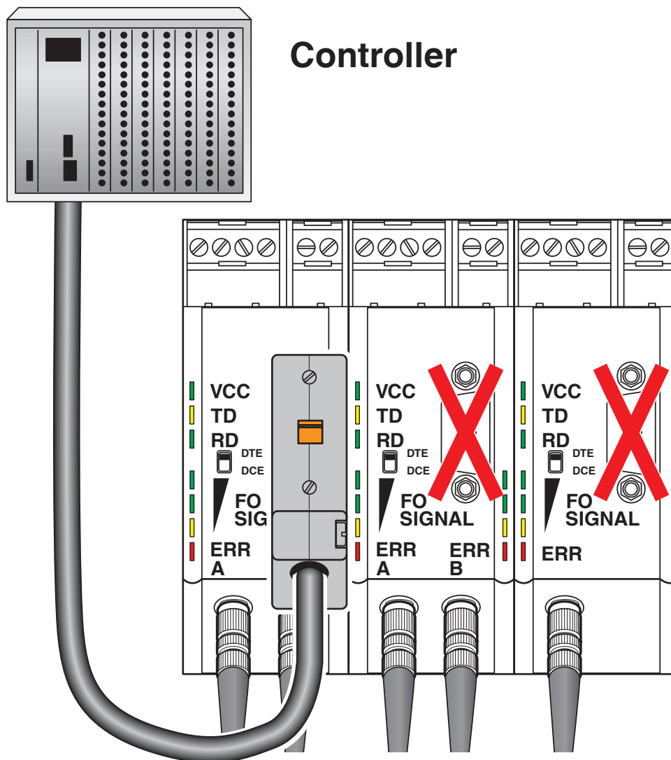
Schemazeichnung
