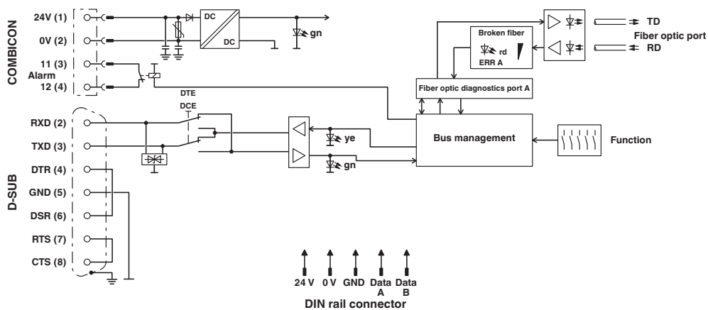
Schéma fonctionnel
