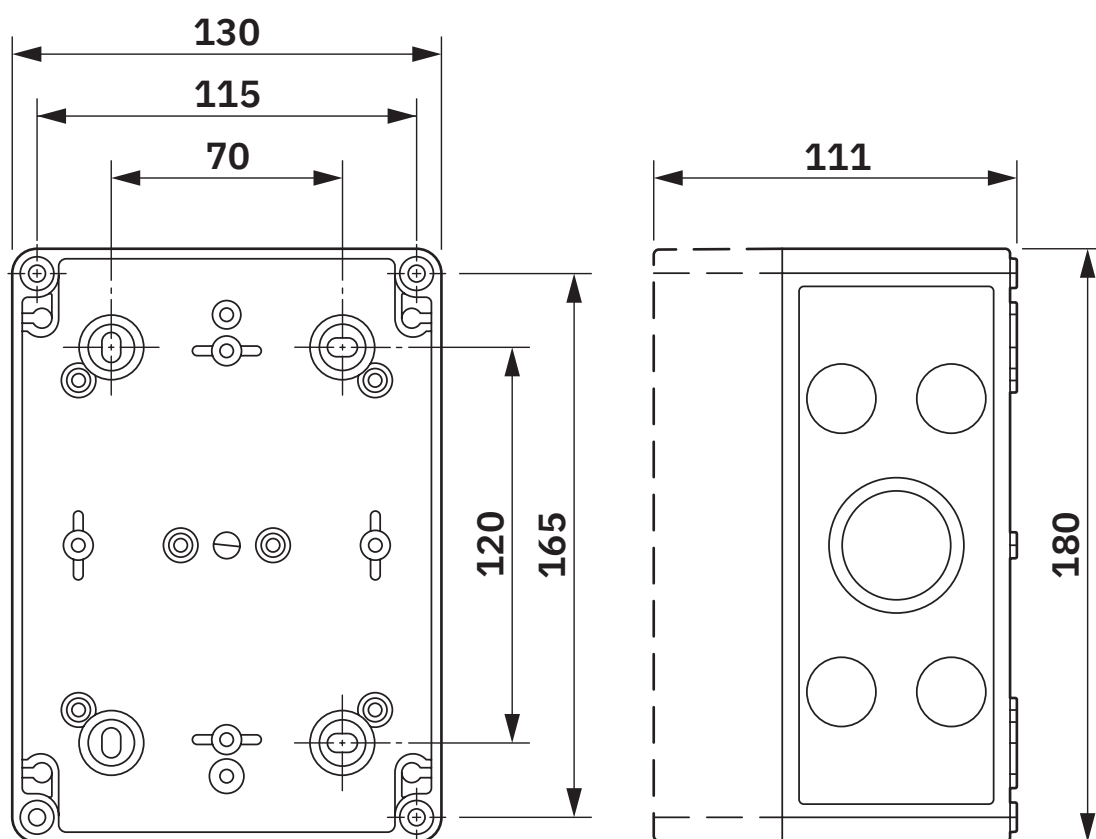
Maßzeichnung
