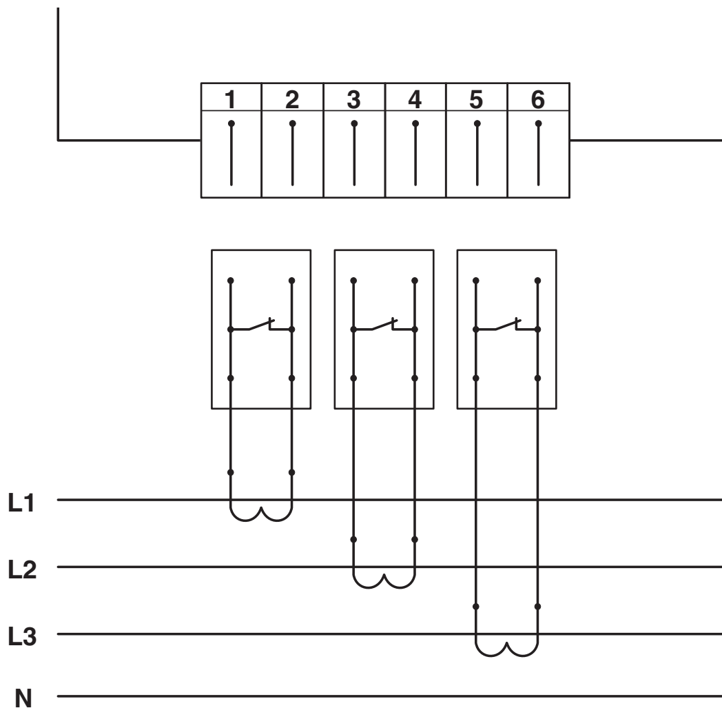
Diagrama eléctrico
