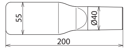
Maßbild FD 60 MS
