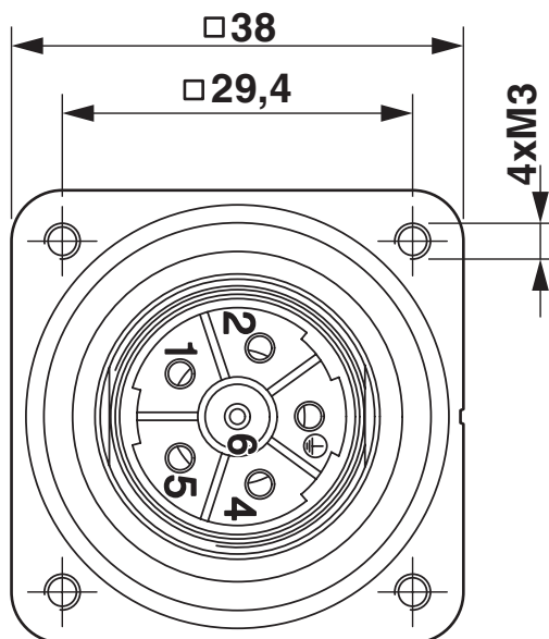
Esquema de dimensiones
