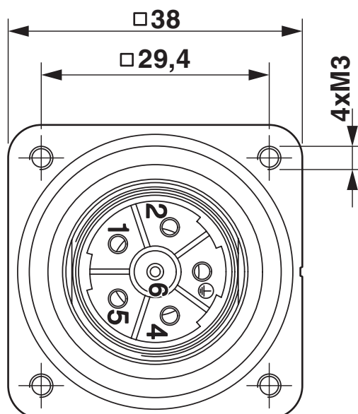
Dessin coté
