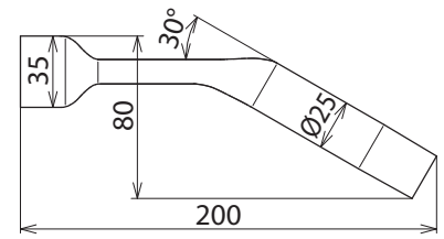
Maßbild QD 35 W NS
