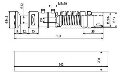
Maßbild AE ISO RIV KF HVI 75 V2A
