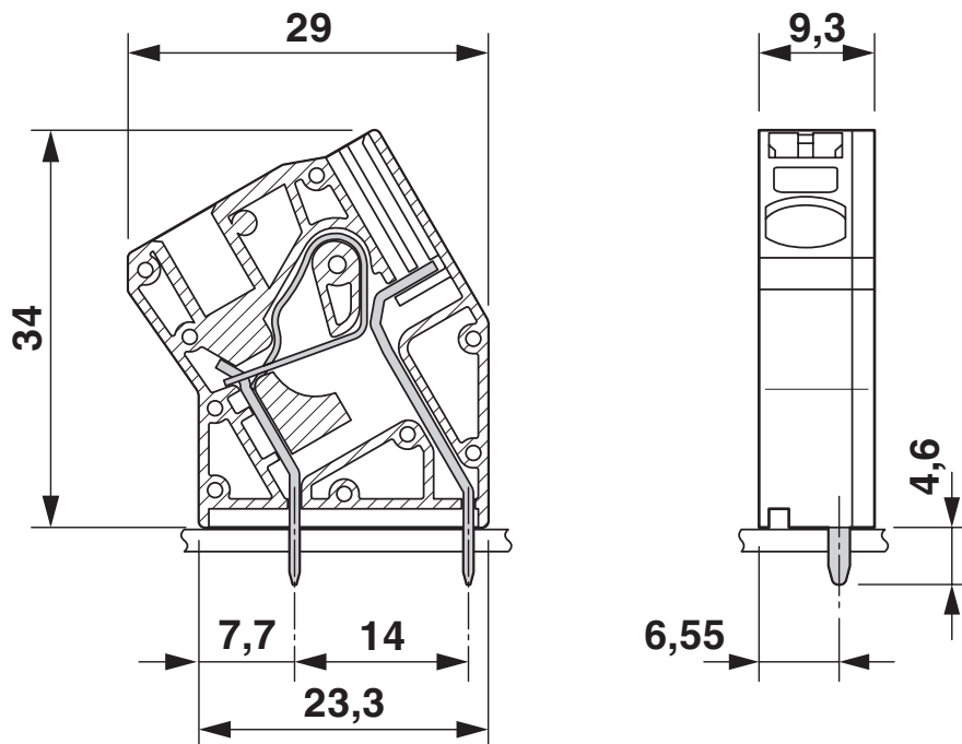
Maßzeichnung
