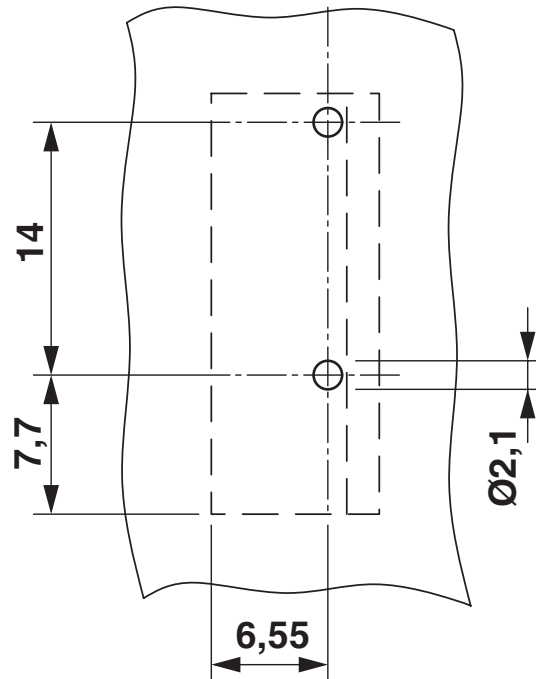
Bohrplan/Lötpadgeometrie
