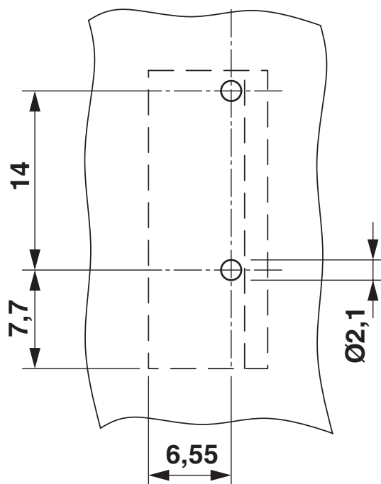
Esquema de taladros/geometría pads soldadura
