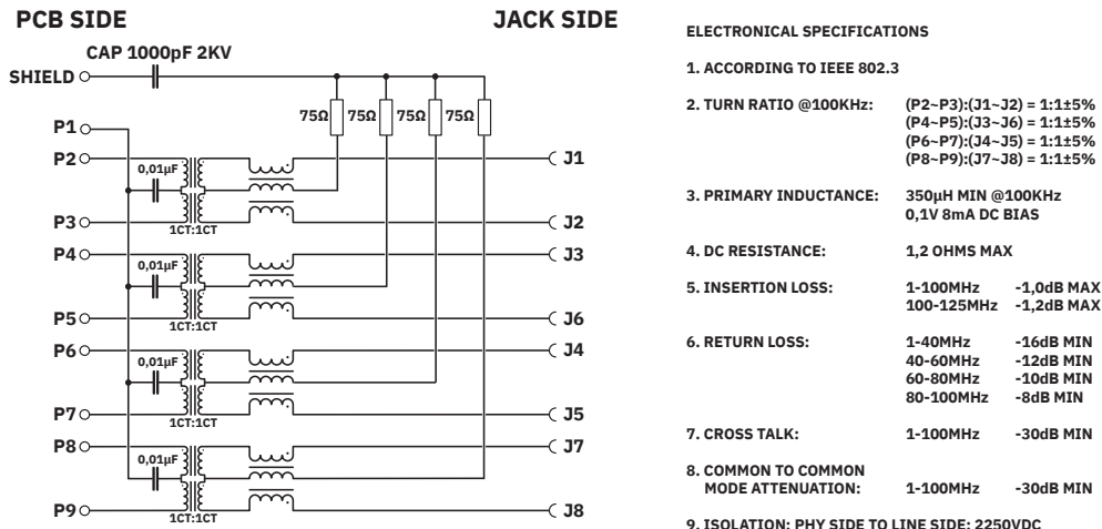
Diagrama eléctrico
