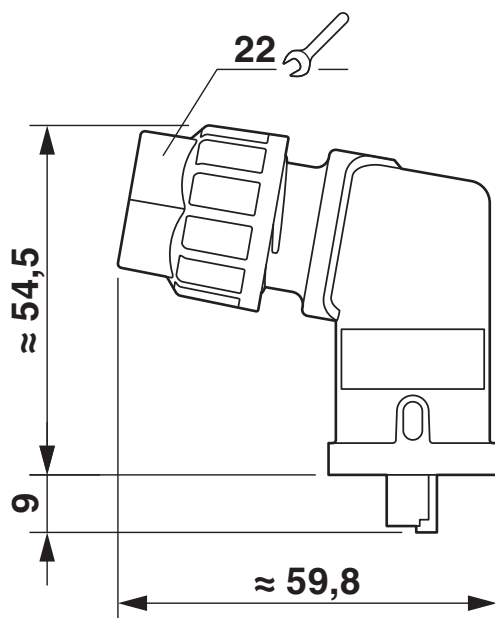
Dessin coté
