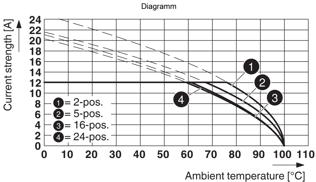
Typ: FRONT-MSTB 2,5/...-ST-5,08 mit MSTBW 2,5/...-G-5,08
