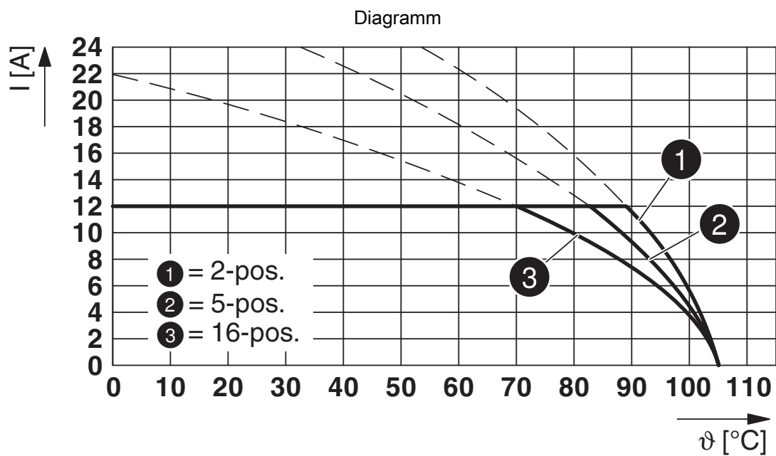
Typ: FKCVR 2,5/...-ST-5,08 mit MSTBW 2,5/...-G-5,08
