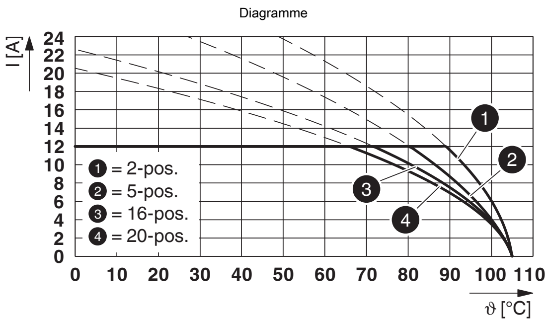
Type : FKCS 2,5/...-ST-5,08 avec MSTBW 2,5/...-G-5,08
