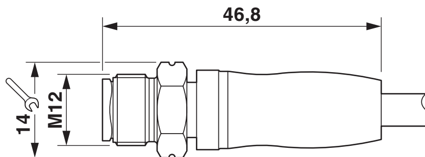
Dessin coté
