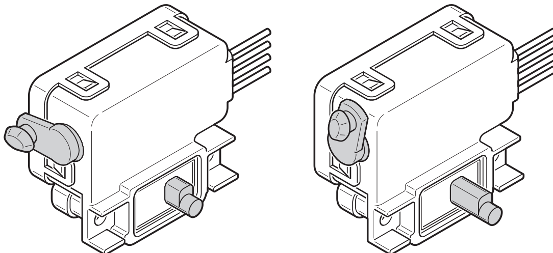
Posiciones de palanca del desbloqueo de emergencia
