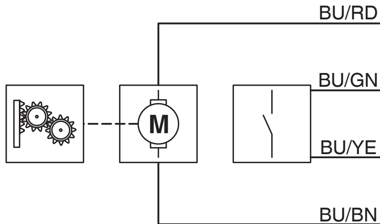
Esquema de conjunto
