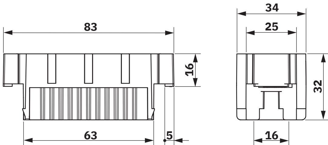
Maßzeichnung
