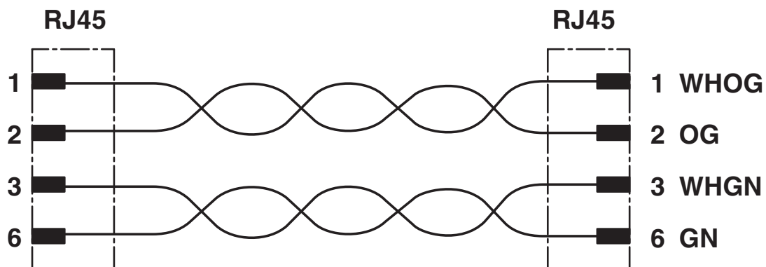
Diagrama eléctrico
