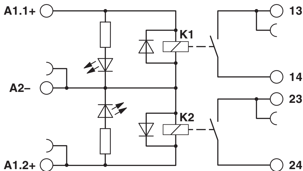
Diagrama eléctrico
