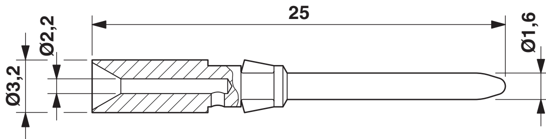
Dessin coté
