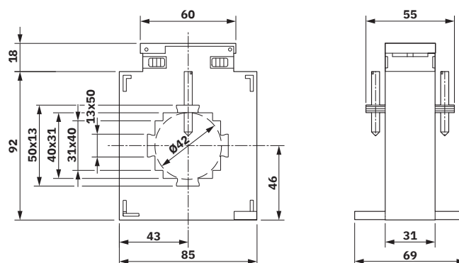
Dessin coté
