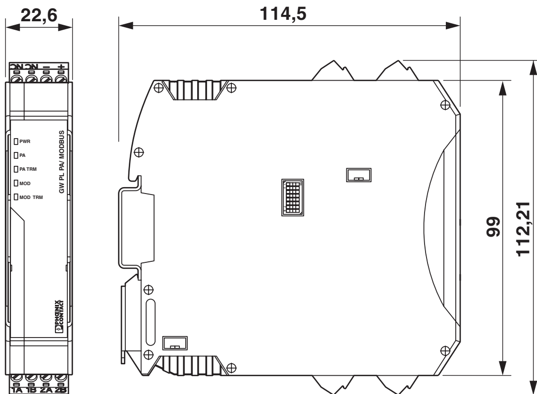
Dessin coté
