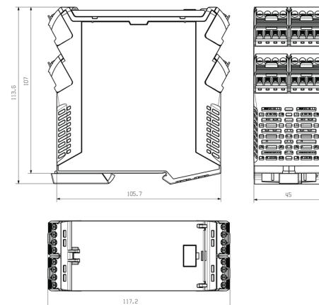
Maßzeichnung
