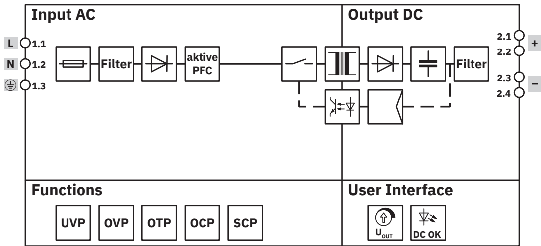
Blockschaltbild
