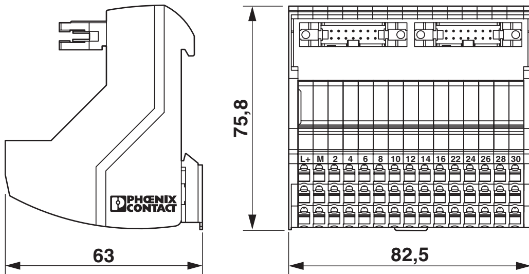
Maßzeichnung
