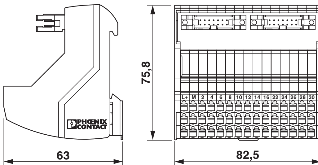
Dessin coté
