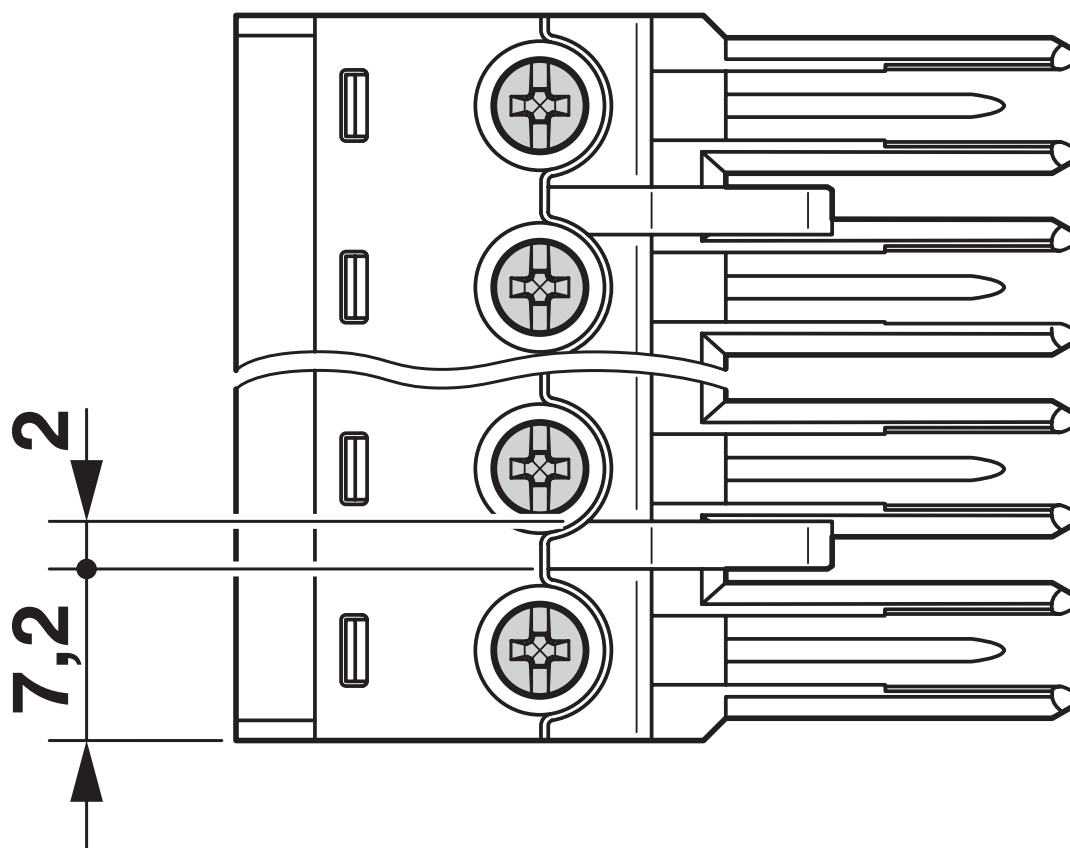
Dessin coté
