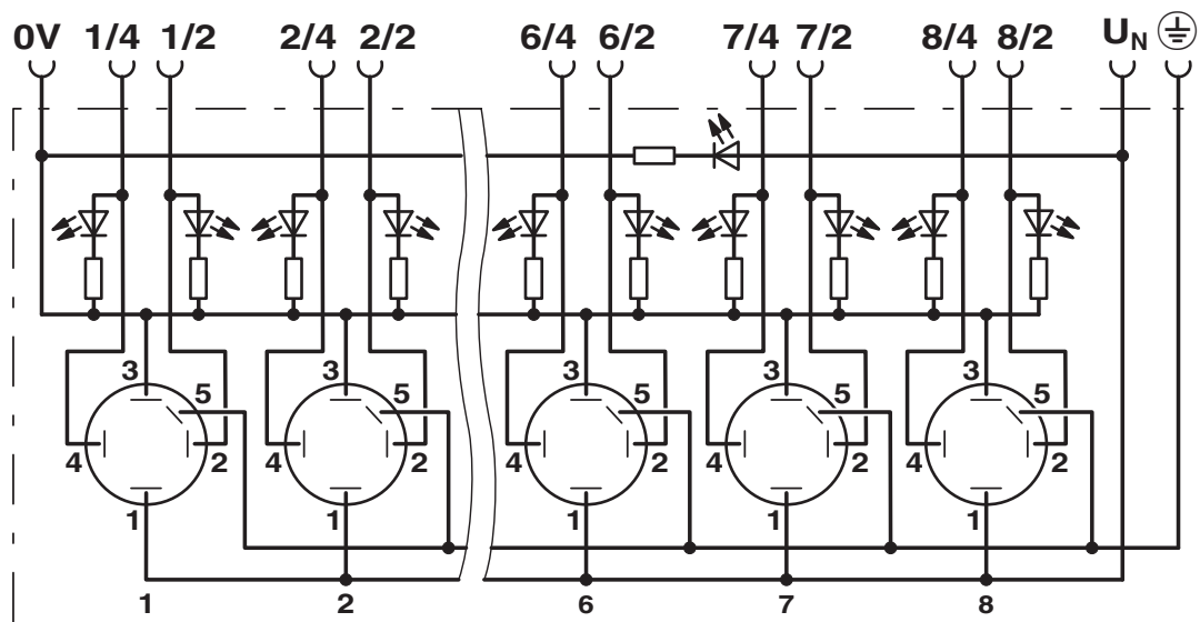
Schaltplan
