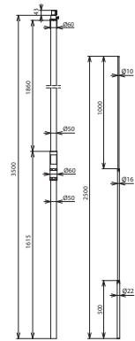
Maßbild SR D50 3500 FS2500 IA HVIP GFK
