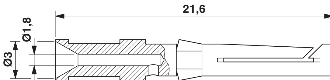
Maßzeichnung
