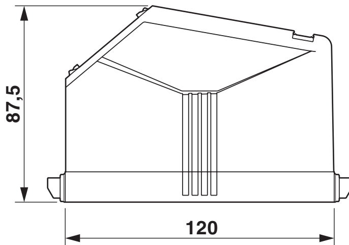
Maßzeichnung
