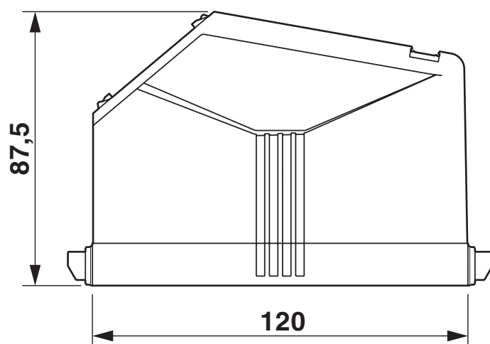
Dessin coté
