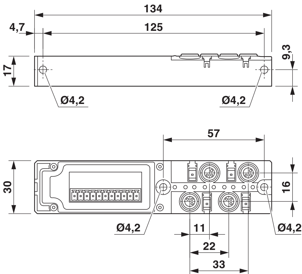
Dessin coté
